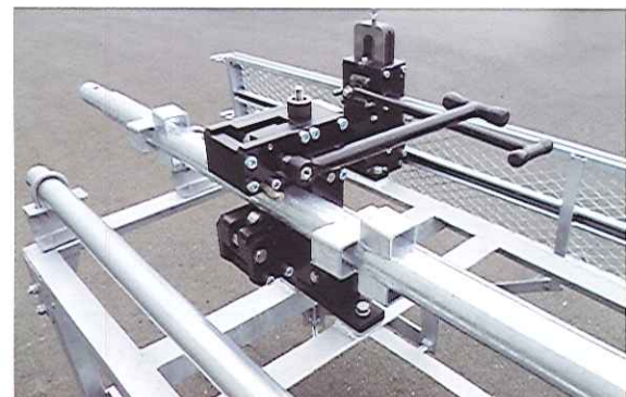
パイプ用刻印機
